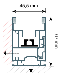
GUÍA ARV COULISSE ARV (HAUTE RÉSISTANCE AU VENT) HWR guide rail (high wind resistance)
