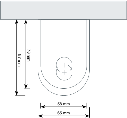
(ES) INSTALACIÓN A TECHO (FR) Installation au plafond (EN) Installation on the ceiling
