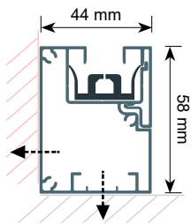
GUÍA ÚNICA COULISSE UNIQUE Única guide rail
