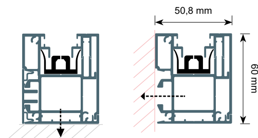
GUÍA SISTEMA TENSIONADO COULISSE SYSTÈME TENDU Tension guide rail system
