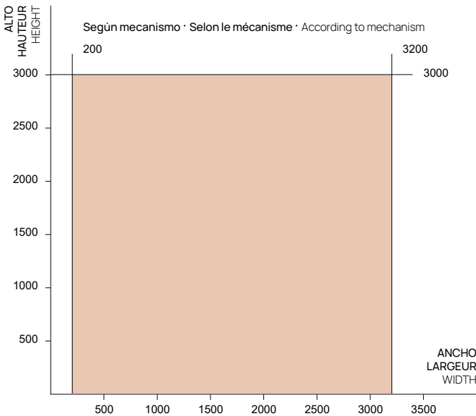
EJE 56 (FR) AXLE · (EN) Axe
