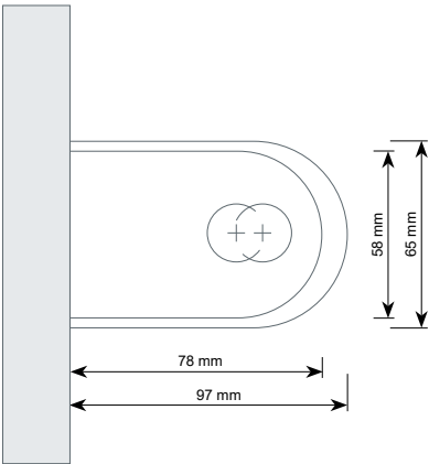
(ES) INSTALACIÓN A PARED (FR) Installation au mur (EN) Installation on the wall
